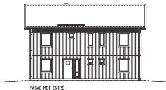
FASAD MOT ENTRÉ
