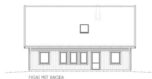
FASAD MOT BAKSIDA
