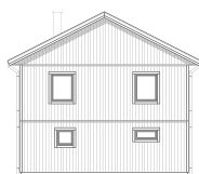
FASAD MOT VÄNSTER
